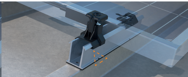
HOOG MONTAGEPROFIEL VOOR PLAATSING OPTIMIZER OF MICRO-OMVORMER
