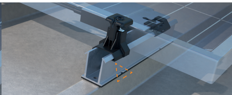
HÖG MONTAGEPROFIL FÖR INSTALLATION AV OPTIMIZER ELLER INSTALLATION AV MIKROINVERTERARE
